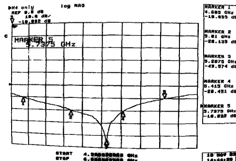
그림 12. 실제 측정된 반사계수
