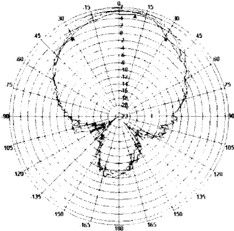
그림 13-b. Elevation 방사패턴
