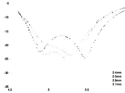
그림 5. 슬롯 X2 변화에 따른 반사계수
