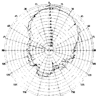
그림 13-a. Azimuth 방사패턴
