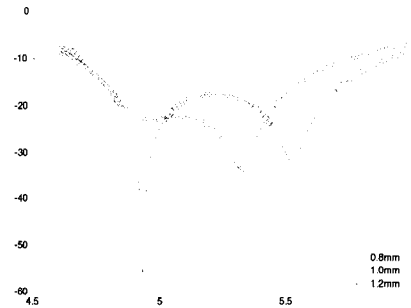
그림 4. 슬롯 Y1 변화에 따른 반사계수
