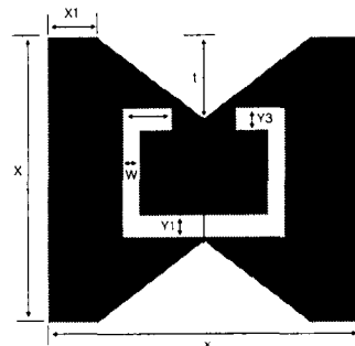
그림 1(a). 설계된 안테나 구조
