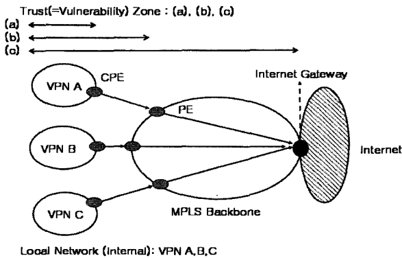
(그림 2) 다중 VPN과 신뢰구역
