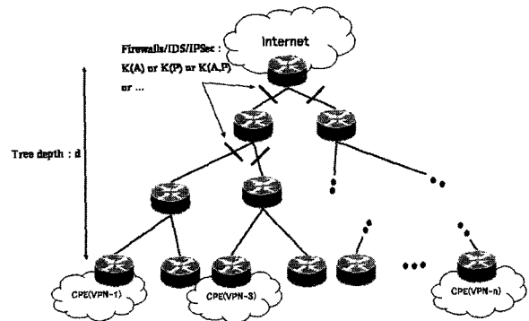
(그림 8) Depth 4의 다중 VPN 네트워크
