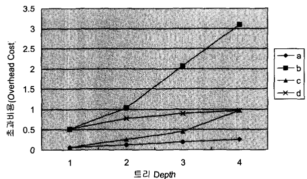
(그림 9) 트리 depth가 4일 경우
