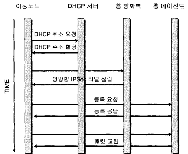
(그림 7) 메시지 교환 단계
