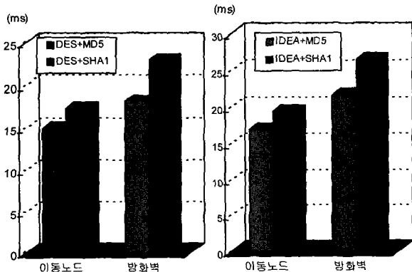
(그림 14) DES 암호 알고리즘과 MD5, SHA-1 해쉬 알고리즘 적용 (Case 4) (그림 15) IDEA 암호 알고리즘과 MD5, SHA-1 해쉬 알고리즘 적용 (Case 4)
