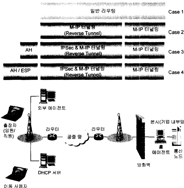
(그림 8) 시뮬레이션 시나리오 및 망 구성
