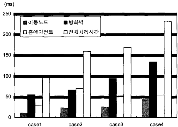
(그림 9) 노드별 평균 처리시간
