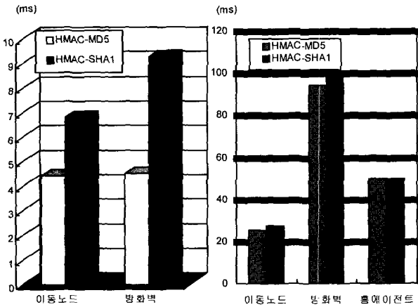
(그림 12) 해쉬 알고리즘 수행시간 비교 (Case 3) (그림 13) AH를 지원하기 위한 노드별 처리시간 (Case 3)
