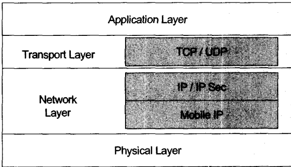
(그림 3) IPSec과 Mobile IP의 통합 구조
