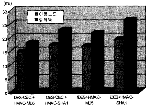
(그림 16) AH, ESP를 지원하기 위한 알고리즘의 수행시간 비교(Case 4)
