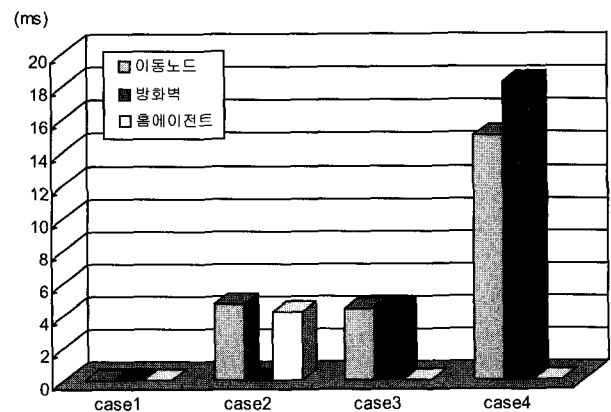
(그림 11) 노드 암호화 시간(등록요청) HMAC-MD5, DES-CBC
