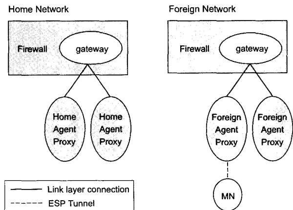
(그림 1) FATIMA 구조도
