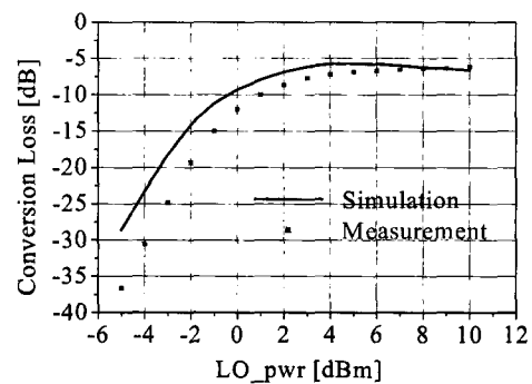
그림 6. 제작된 혼합기의 LO 전력에 따른 변환 손실 곡선 Fig. 6. LO characteristics of the manufactured mixer.
