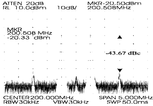
그림 9. 제작된 혼합기의 3차 상호 왜곡 신호의 출력 스펙트럼(LO frequency = 2 GHz, LO power = 6 dBm, RF power = -14 dBm, IF1 = 200.5 MHz, IF2 = 199.5 MHz)
