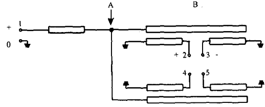
그림 2. Microstrip과 CPS를 이용한 새로운 발룬회로 Fig. 2. A novel balun using microstrip to CPS.
