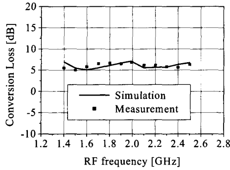
(a) 주파수 하향 변환기 (a) Downconverter
