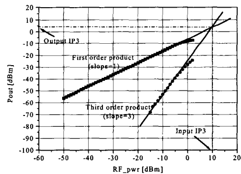
그림 8. Extrapolation을 이용한 혼합기의 TOI 계산 Fig. 8. TOI calculation of the mixer using extrapolation.
