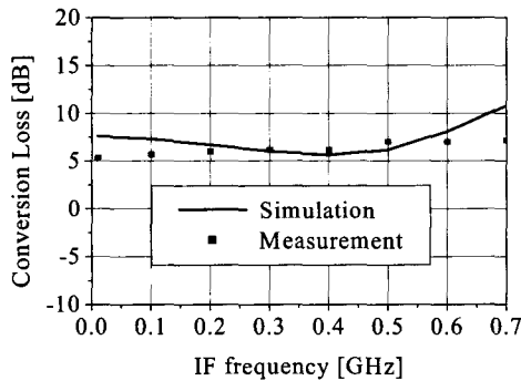
(b) 주파수 상향 변환기 (b) Upconverter
