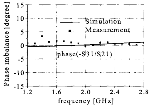
(b) 위상 불평형 정도 (b) Phase imbalance
