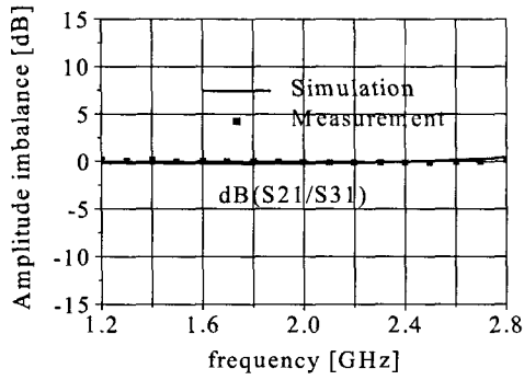
(a) 진폭 불평형 정도 (a) Amplitude imbalance
