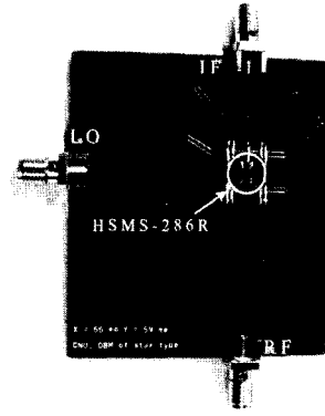
그림 5. 제작된 이중 평형 혼합기의 사진 Fig. 5. The photograph of the manufactured double balanced star mixer.
