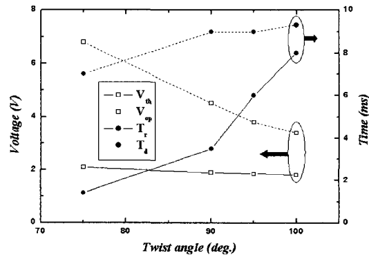
그림 4. Twist angle에 따른 rising time과 decay time, 문턱전압 그리고 구동전압에 대한 그래프.
