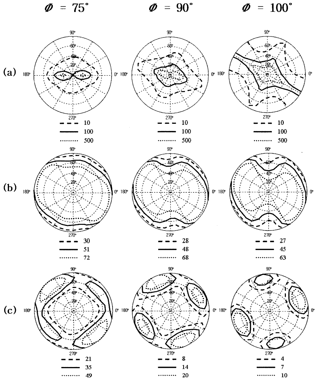
그림 5. (a) Twist angle에 따른 등 명암 대비율 곡선. (b) Twist angle에 따른 전압 무인가시 등 반사율 곡선. (c) Twist angle에 따른 전압 인가시 등 반사율 곡선. Fig. 5. (a) Iso-contrast contour for twist angles. (b) Iso-reflectance contour at off-state for twist angles. (c) Iso-reflectance contour at on-state for twist angles.
