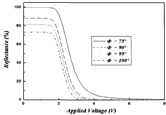
그림 3. 입사 파장이 550nm에서 액정의 twist angle에 따른 전압에 따른 반사율 곡선.
