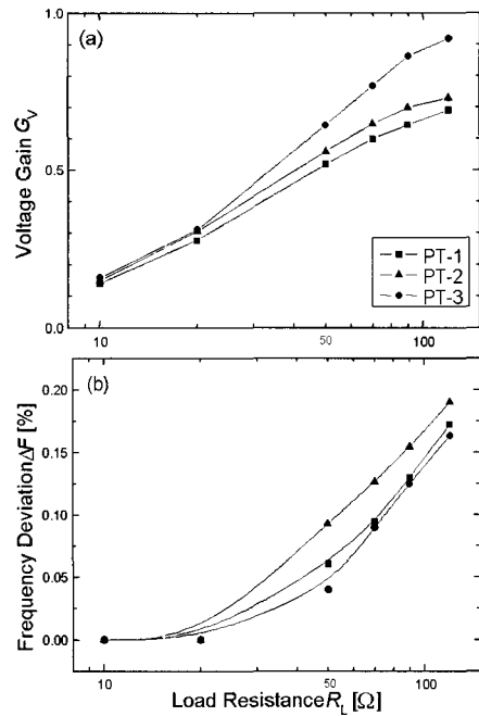
그림 5. 부하저항에 따른 (a) 전압이득 및 (b) 주파수 편이량의 상관관계.
