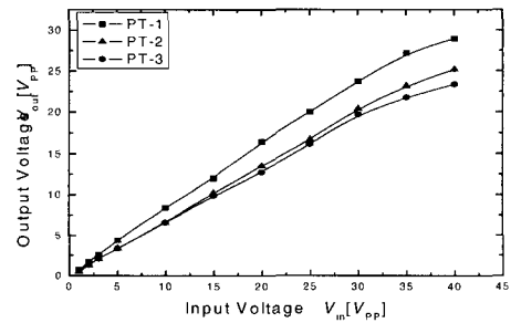
그림 6. 입력 및 출력전압의 상관관계.
