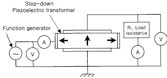
그림 2. 감압용 압전 변압기의 측정회로. Fig. 2. Circuit for the characterization of step-down piezoelectric transformer.
