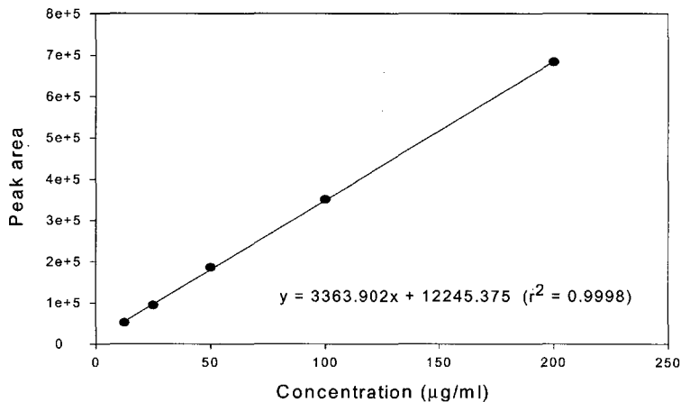
Fig. 1. Matrine의 표준검량선
