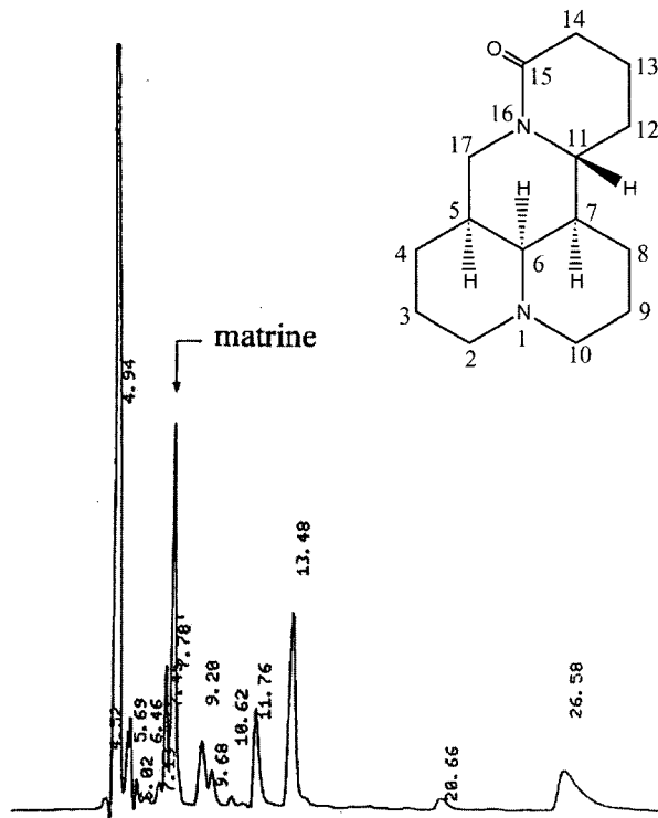
Fig. 2. 고삼 alkaloid 분석의 HPLC chromatogram (GS-34)
