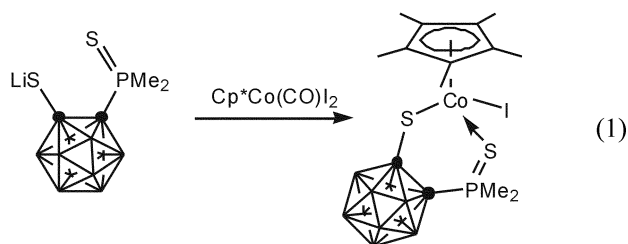
LiS(S=PMe 2 )C 2 B 10 H 10 ( 2b ) Cp*CoI[S,S'-S(S=PMe 2 )C 2 B 10 H 10 ]( 4 )
