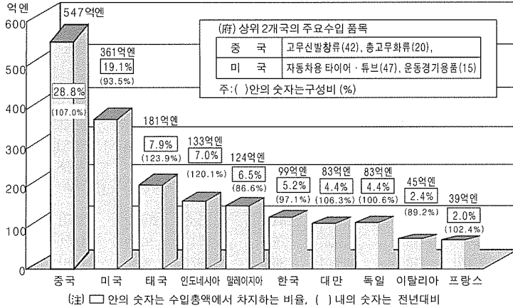
고무 제품의 주요수입국 (2002년도)
