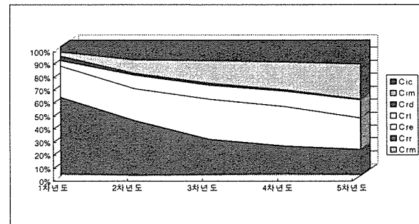
그림 15. 비용분해항목 프로파일
