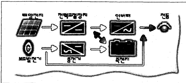
그림 3 태양광 발전 시스템의 구성도
