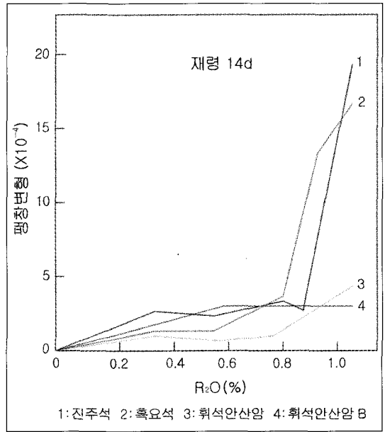
〈그림-4〉 시멘트 중의 알카리 양과 몰탈의 팽창과의 관계
