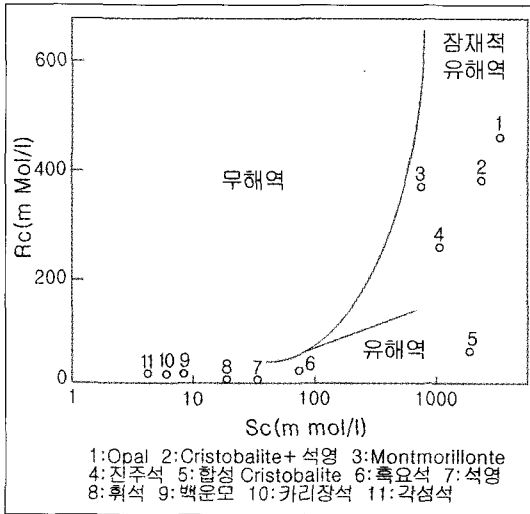
〈그림-3〉 Rc와 Sc와의 관계
