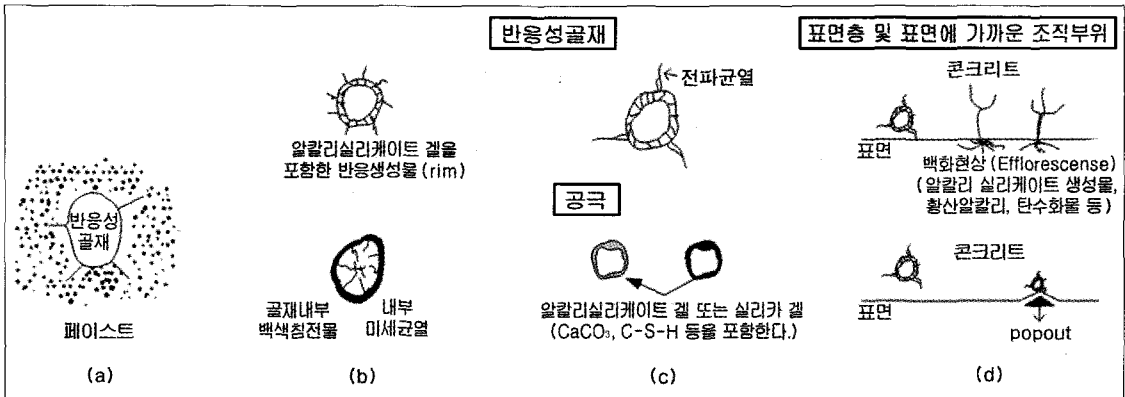
〈그림-1〉 알카리골재반응의 진행 모델의 예
