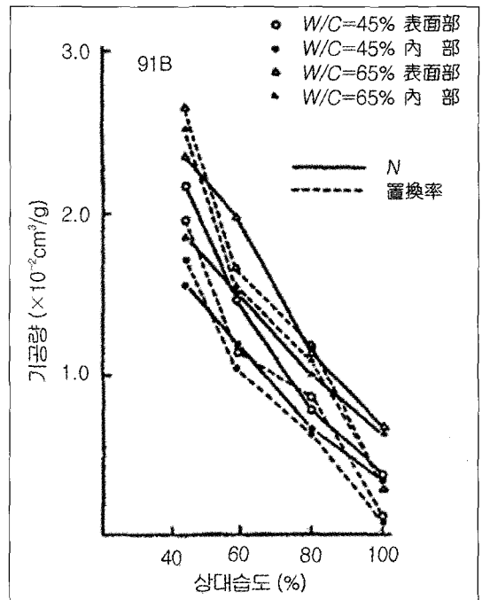
〈그림-7〉 상대습도와 세공량의 관계
