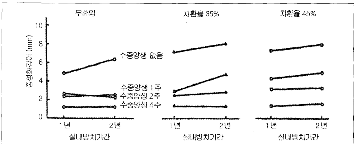
〈그림-8〉 초기양생 기간의 차이가 중성화에 미치는 영향
