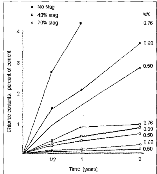
〈그림-3〉 시간에 따른 염소이온의 함량
