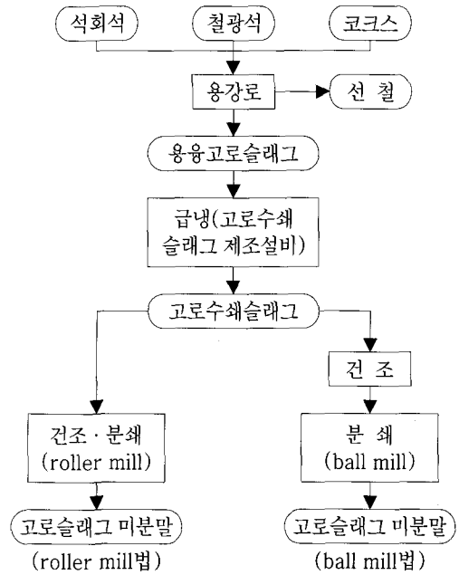
<그림-1> 고로슬래그 미분말의 제조 과정
