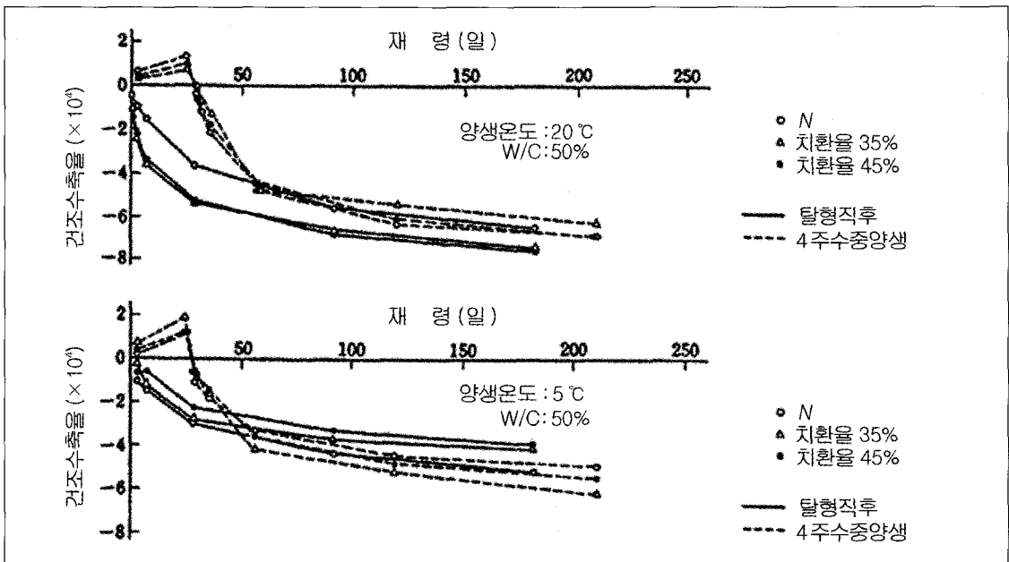
〈그림-10〉 재령과 건조수축율의 관계
