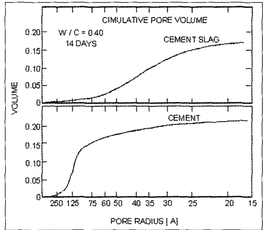
〈그림-2〉 공극 크기 분포도
