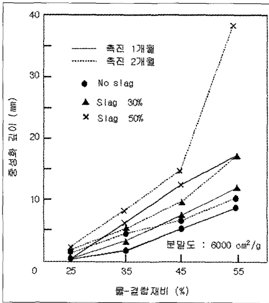
〈그림-6〉 콘크리트의 중성화 시험결과
