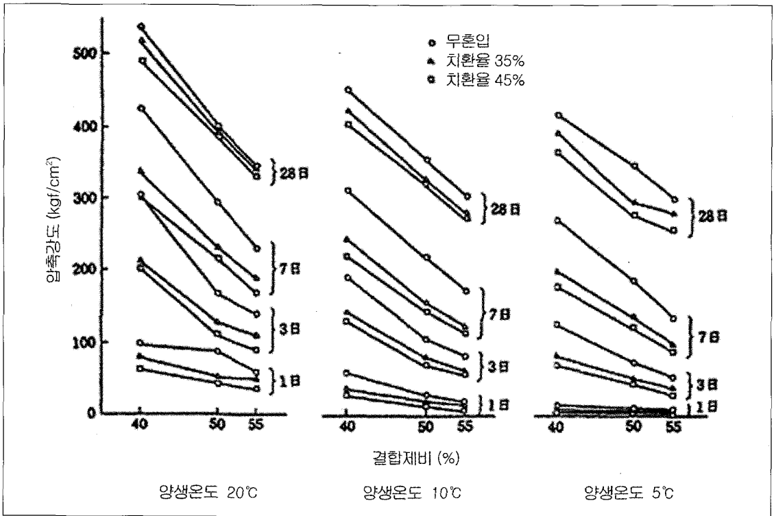
〈그림-5〉 양생온도와 압축강도의 관계
