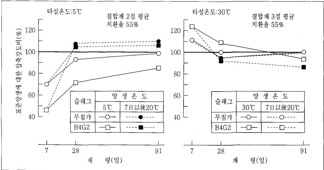
〈그림-4〉 재령별 표준양생에 대한 압축강도비의 관계
