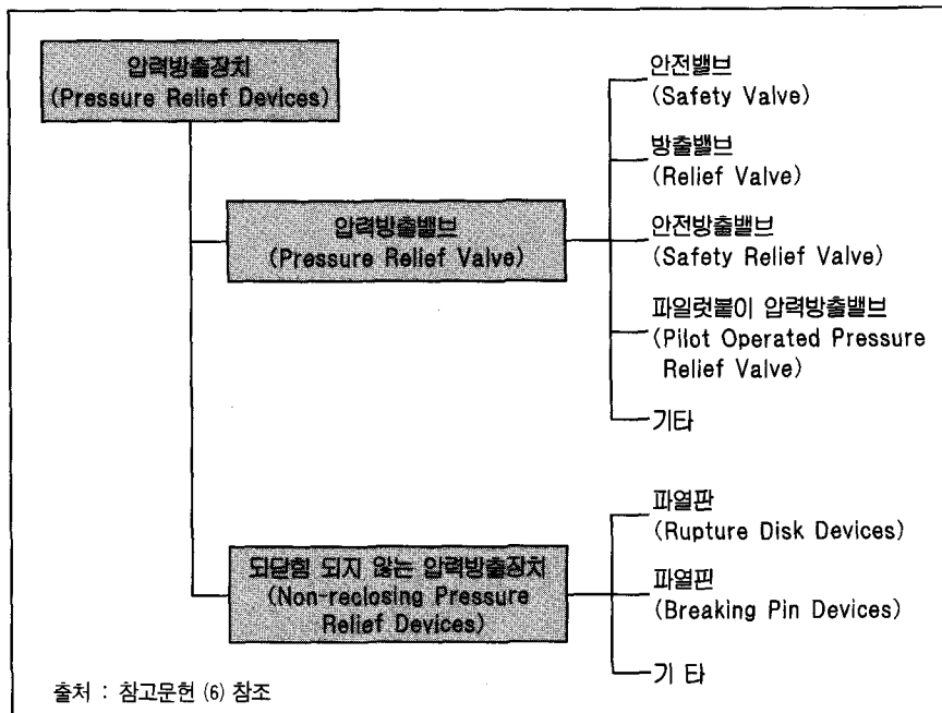
〈그림 1〉 압력방출장치의 종류
