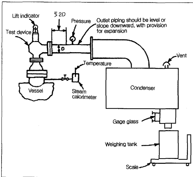
〈그림 3〉 응축수 중량 시험법
