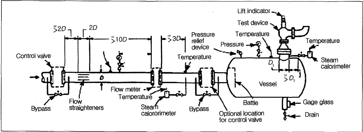
〈그림 2〉 유량계 시험법
