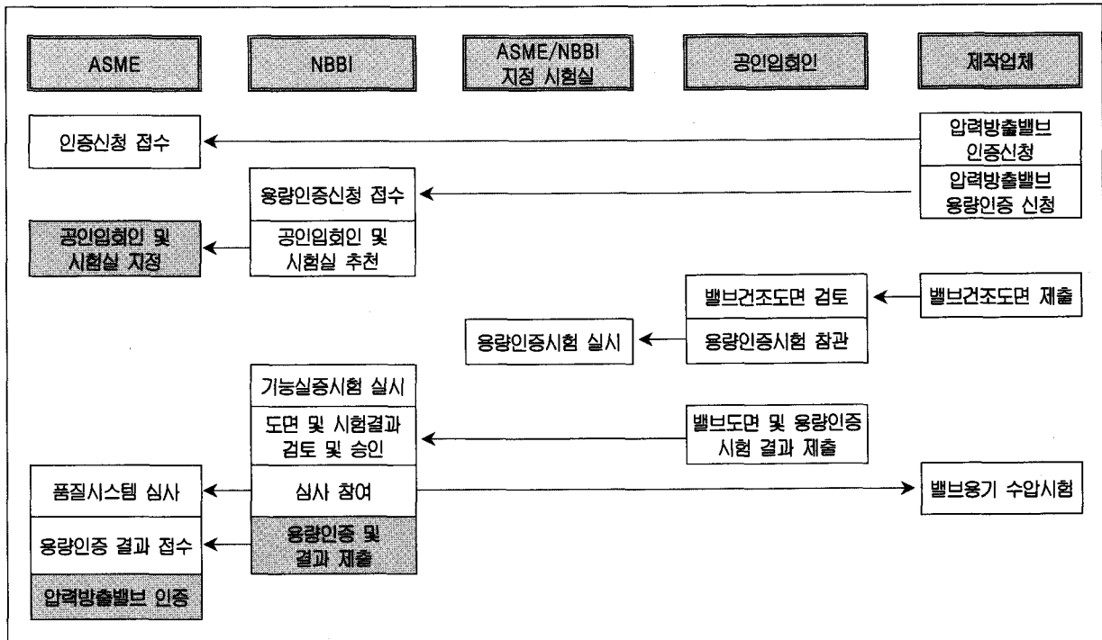
〈그림 4〉 ASME Sec. III 압력방출밸브의 인증절차
