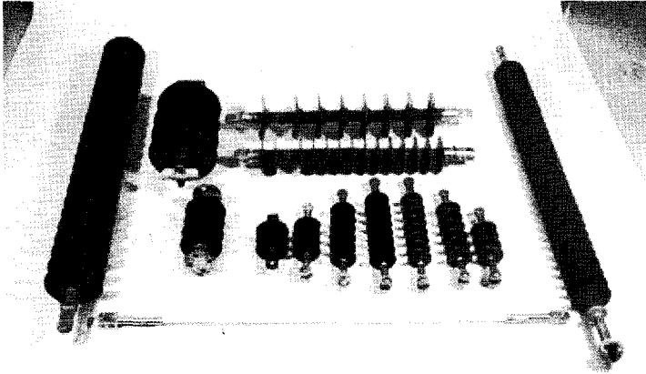
〈송배전용 폴리머애자〉
