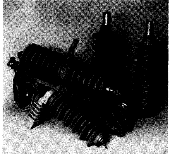
〈폴리머 COS-피뢰기-부싱〉
