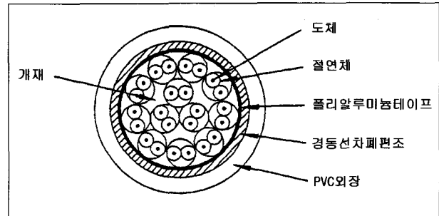
〈그림 21〉 GP-IB케이블의 구조 예
