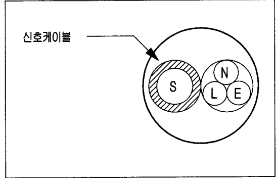
〈그림 25〉 신호선을 포함한 복합형기기케이블
