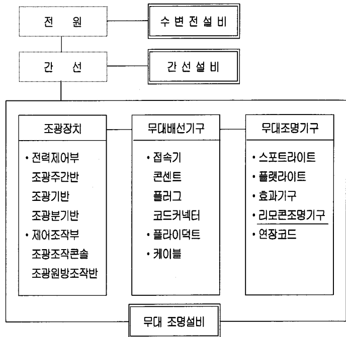
〈그림 1〉 무대 조명설비의 구성
