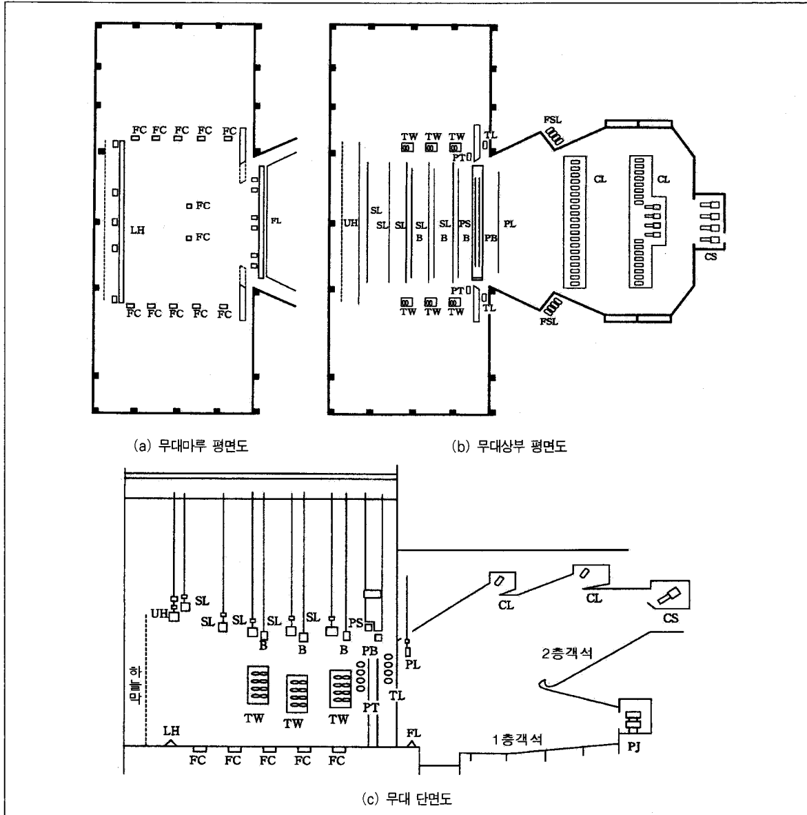
<그림 2> 무대조명기구 배치도의 일례
