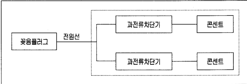
〈그림 15〉 분기콘센트박스의 구성도
