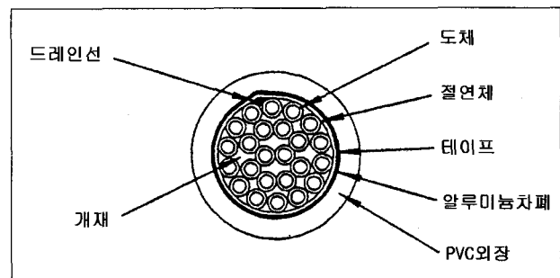
〈그림 22〉 컴퓨터용 다심케이블의 구조 예
