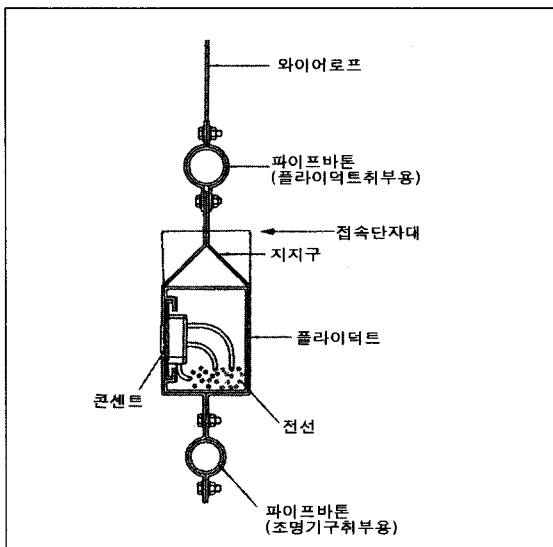
〈그림 16〉 콘센트식 플라이덕트
