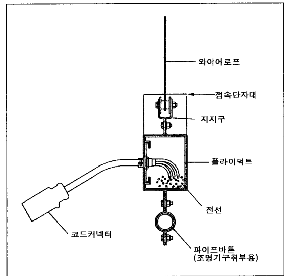
〈그림 17〉 커넥터식 플라이덕트
