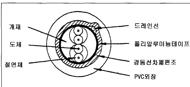
〈그림 20〉 RS-422, RS-485 케이블의 구조 예
