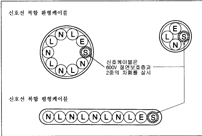
〈그림 24〉 신호선을 포함한 복합형보더케이블
