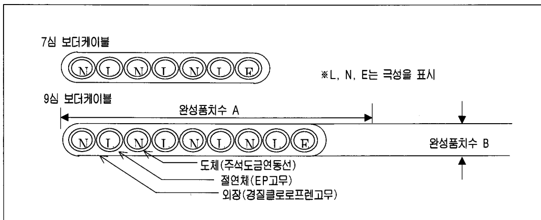
〈그림 19〉 평형 보더케이블의 구조 예
