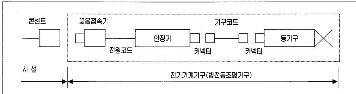
〈그림 8〉 방전등조명기구(안정기 분리형)
