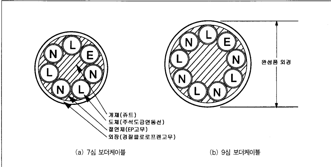
〈그림 18〉 환형 보더케이블의 구조 예
