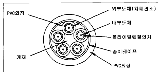
〈그림 23〉 동축다심케이블의 구조 예
