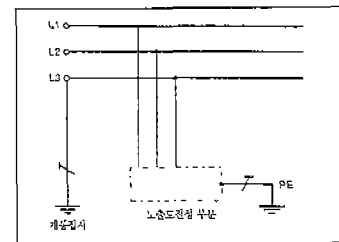
그림6 TT 계통
