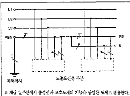
그림5 TN-C 계통
