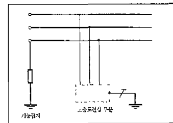
그림7 IT 계통
