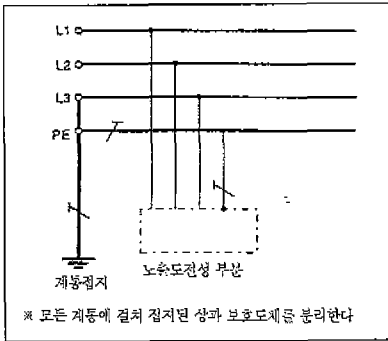
그림3 TN-S 계통
