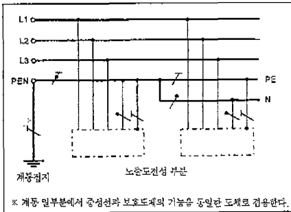
그림4 TN-C-S 계통
