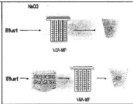
그림6. Fouling제어방법(上;NaOCl, 下; 응집/침전)
