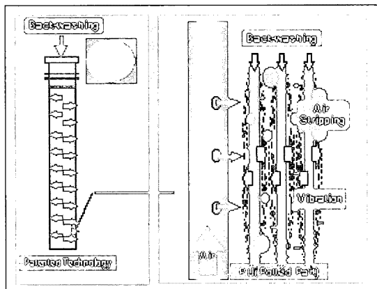
그림2. VSA(Vibrating and Stripping by Air)의 원리
