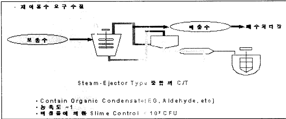
그림4. STEAM EJECTOR 형 폴리에스테르중합공정 냉각탑과 요구수질
