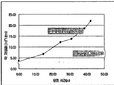
그림5. 응집/침전 전처리효과
