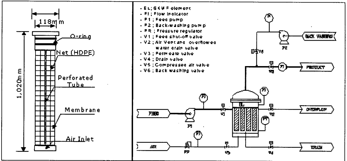
그림3. VSA사양과 장치구성도
