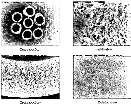
그림1. VSA SYSTEM에 적용되는 분리막의 전자현미경사진
