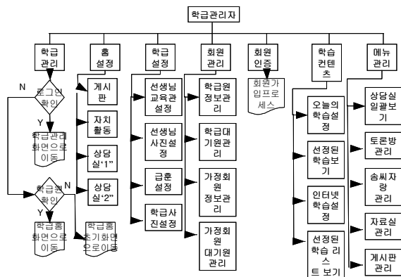
<그림 6> 학급 관리자 모듈 흐름도
