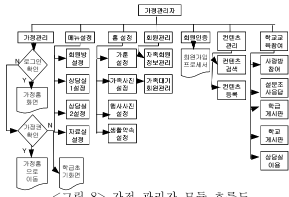
<그림 8> 가정 관리자 모듈 흐름도
