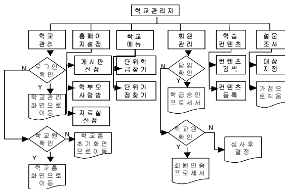
<그림 4> 학교 관리자 모듈 흐름도
