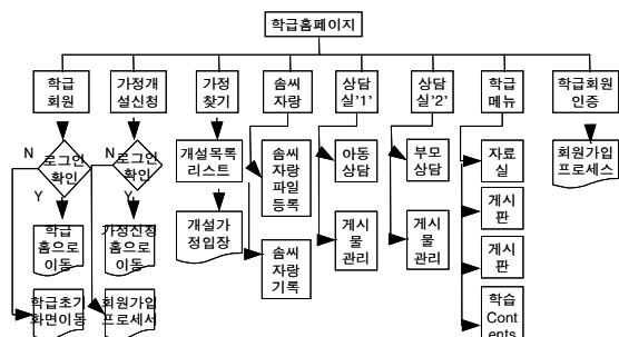
<그림 7> 학급 사용자 모듈 흐름도
