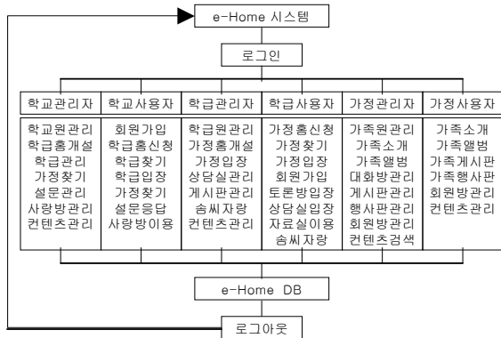
<그림 3> e-Home시스템 모듈 구성도
