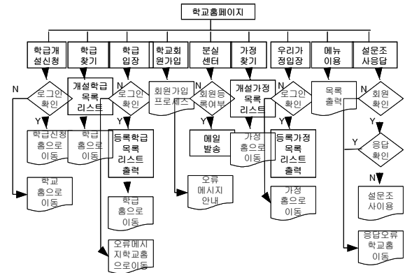
<그림 5> 학교 사용자 모듈 흐름도
