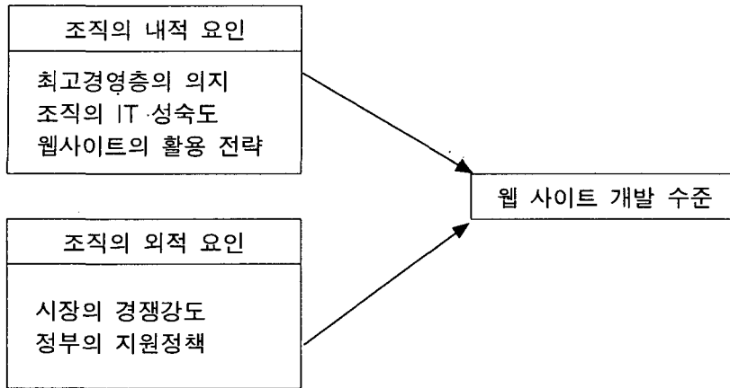
<그림 1> 연구모형
