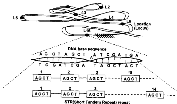
(그림 1) The STR information of DNA
