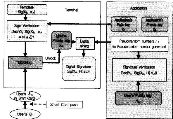
(그림 6) 네트워크에서의 터미널 로그인 다중 사용자 인증시스템
