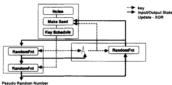
(그림 4) 안전한 의사난수 발생기 구조
