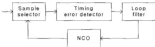
(그림 1) Code tracker의 구성도
