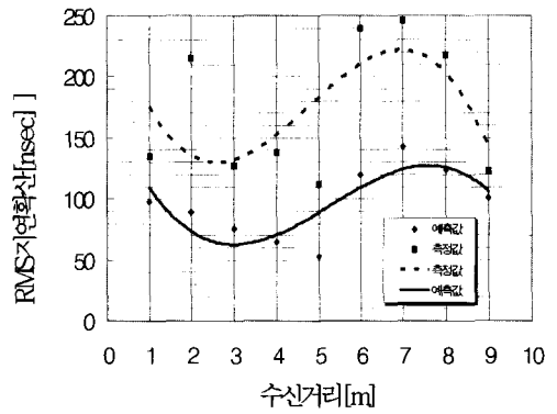
그림 8. 주거지역에서 LOS의 예측·측정 RMS 지연확산 비교
