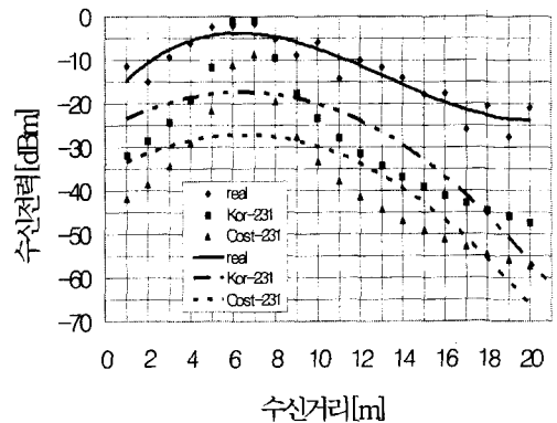
그림 3. 공업지역의 LOS에서 수신전력 비교
