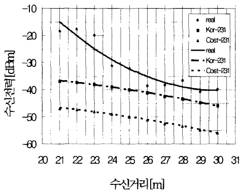
그림5. 공업지역에서 N-LOS의 예측·측정 수신전력비교
