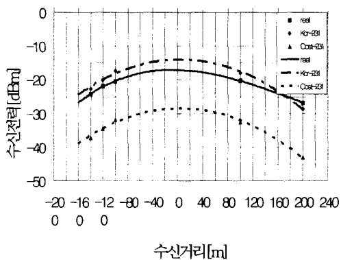
그림6. 주거지역에서 N-LOS의 예측·측정 수신전력비교
