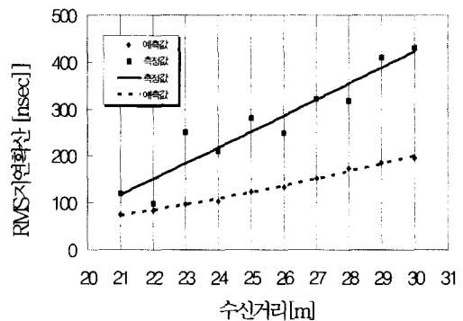
그림 9. 공업지역에서 N-LOS의 예측·측정 RMS 지연확산 비교
