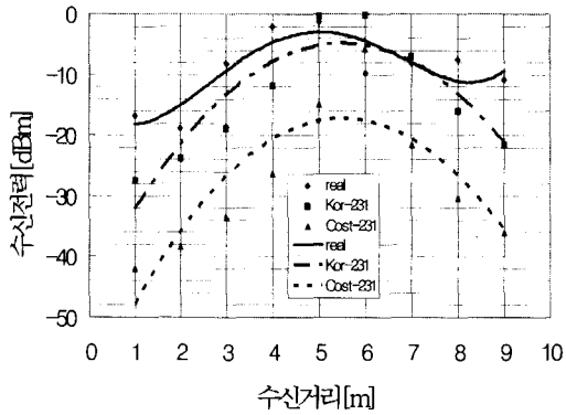
그림 4. 주거지역의 LOS에서 수신전력 비교
