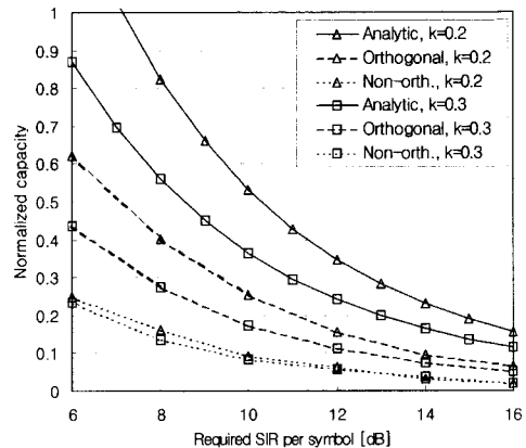
그림 7. 직교 코드 간섭 인자가 0.2와 0.3 일 경우 요구 SIR에 따른 빔 용량.
