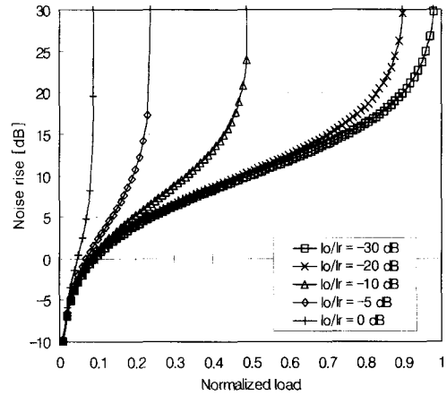
그림 10. 빔 부하에 따른 빔 수신 전력과 잡음 전력의 비 ( x_{oc}=0.1 ).
