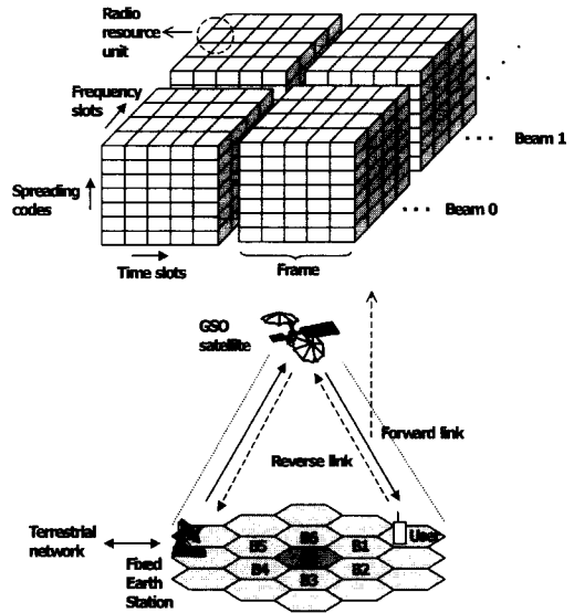
그림 4. 다중빔 위성시스템과 하향링크 전송프레임의 구성.
