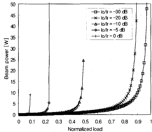
그림 4. 빔 부하에 따른 요구 빔 전송 전력 ( x_{oc}=0.1 ).
