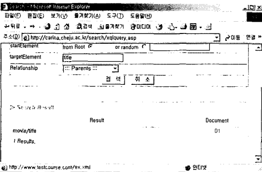
(그림 5) 구조 + 내용 질의 결과
