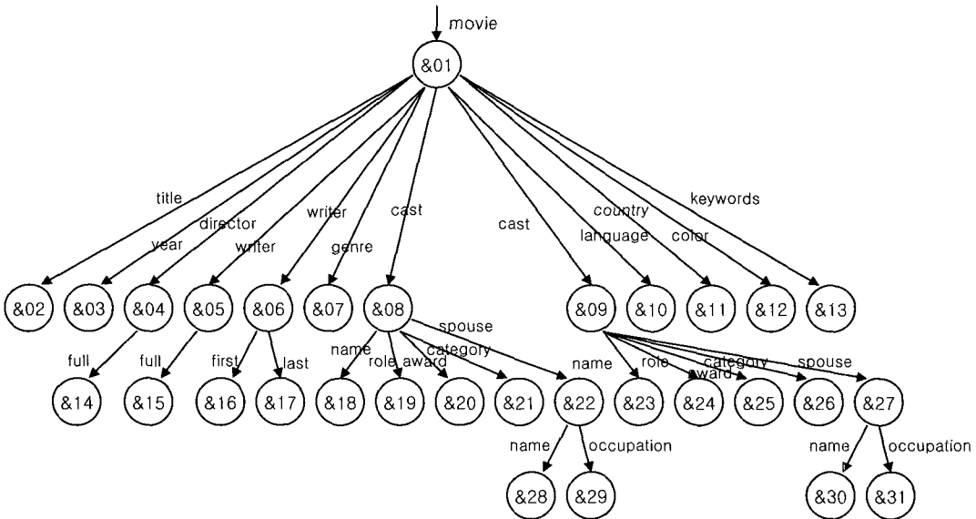
(그림 2) XML 인스턴스에 대한 데이터 그래프(Data Graph)
