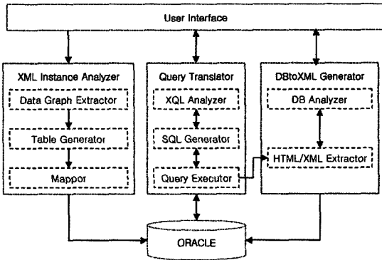
(그림 1) 저장 시스템 구조
