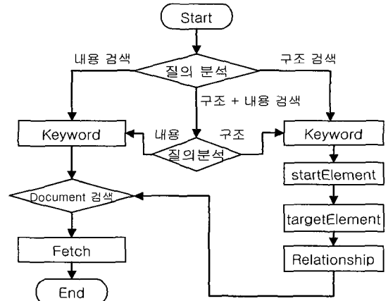
(그림 3) 검색 과정
