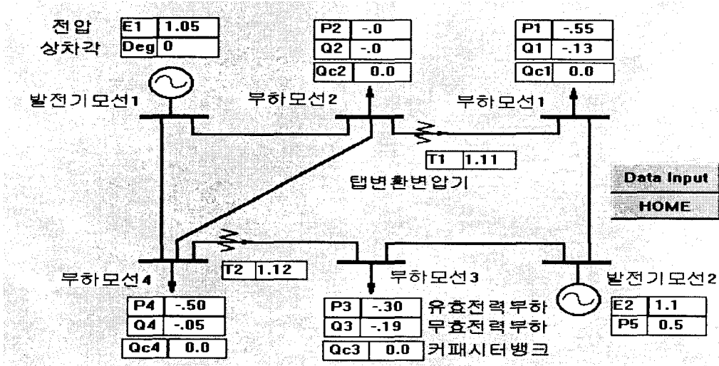
[그림3.] Input Data 화면
