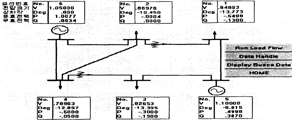
[그림6.] 선로의 조류 화면
