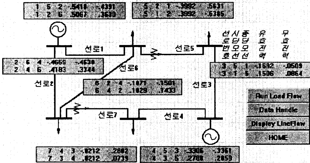
[그림4.] 선로의 상정사고 분석화면
