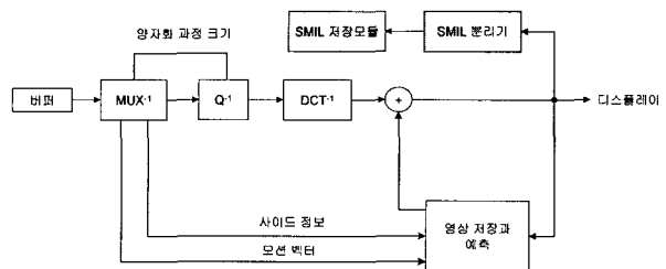
(그림 6) 수정된 MPEG 복호기
