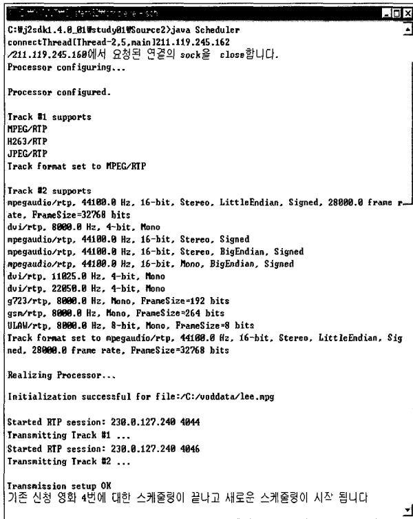
(그림 5) 서버 프로그램과 스케줄러 실행 화면
