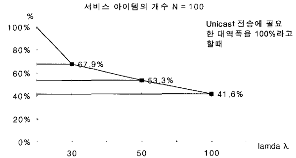
(그림 9) 서비스 요청율에 의한 전송대역폭
