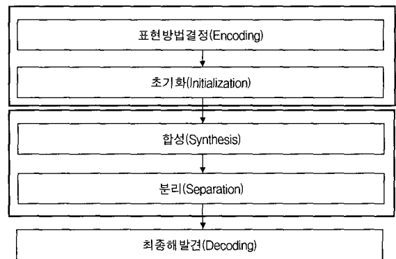
(그림 2) Adleman의 DNA 컴퓨팅 알고리즘
