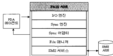
(그림 8) PAIS Server의 구조
