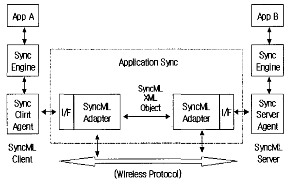
(그림 2) SyncML 프레임 워크 구조도
