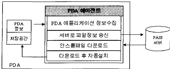
(그림 5) PDA Agent의 구조
