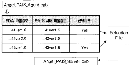
(그림 9) 설치파일 매핑테이블 관리 사례
