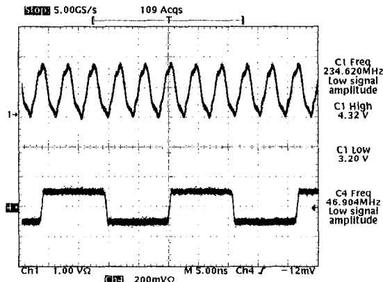
그림 5. 234.7 MHz 클럭 발생기의 입출력 특성
