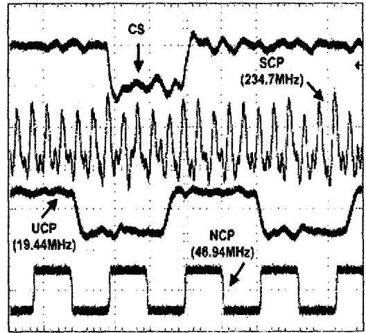
그림 6. 전체 칩의 측정 입출력 특성
