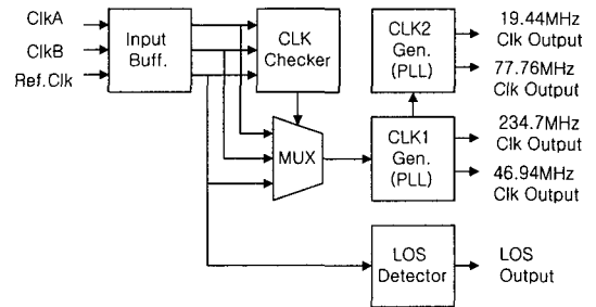
그림 1. 설계된 FMD ASIC의 블록도
