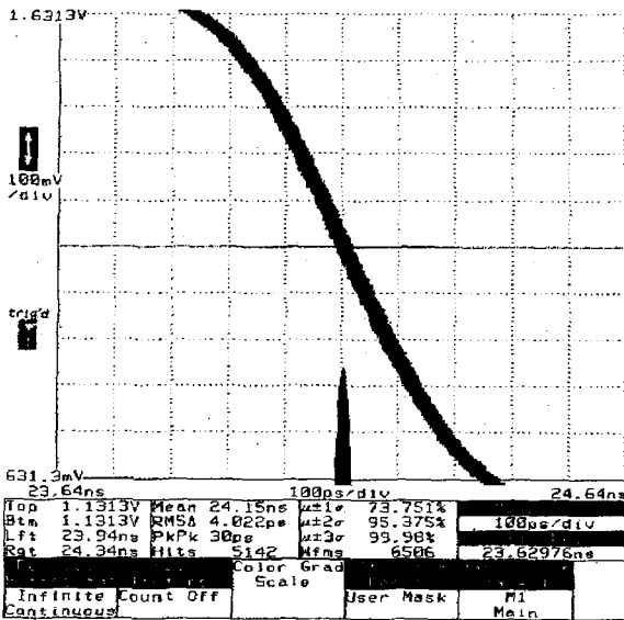
그림 7. 234.7 MHz 클럭의 지터 특성
