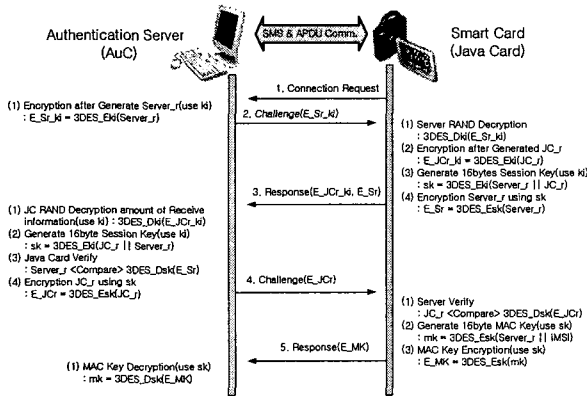
(그림 7) 서버/단말기/자바카드간의 기기인증 및 세션 키 설정 프로토콜
