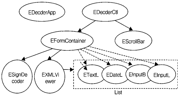
(그림 10) M-EDecoder 모듈의 실행 시간의 객체 구성도
