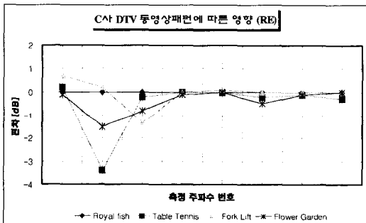
[그림 13] B사와 C사 모델의 동영상 패턴에 따른 RE 레벨의 차이
