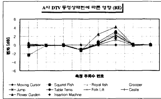
[그림 12] A사 디지털 TV의 동영상 패턴에 따른 RE 레벨의 차이
