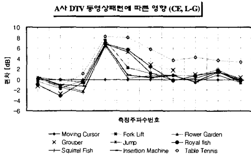
[그림 10] A사 디지털 TV의 동영상 패턴에 따른 CE 레벨의 차이
