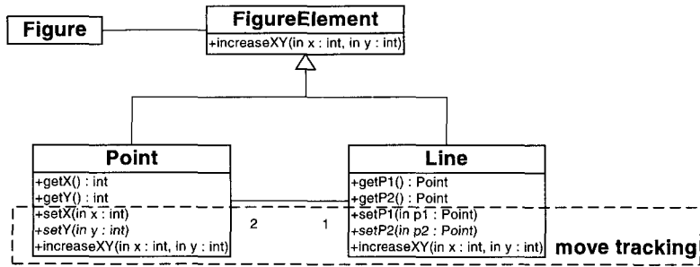
그림 1 간단한 그림 편집기 예제
