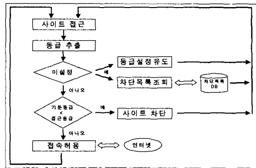
그림 6. 알고리즘 동작흐름도
