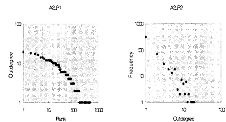
(b) 알고리즘 A2
