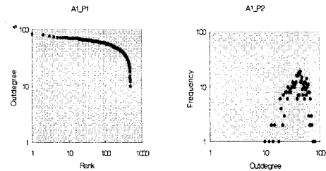
(a) 알고리즘 A1
