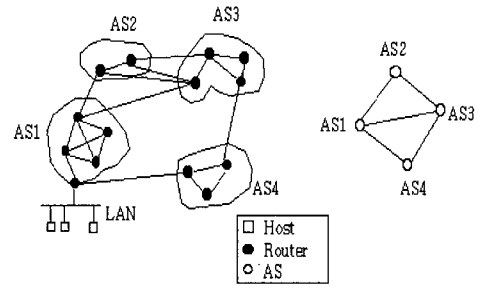
(a) 라우터 계층 (b) AS 계층 그림 1. 인터넷 위상
