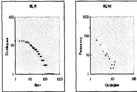
(c) 알고리즘 B3
