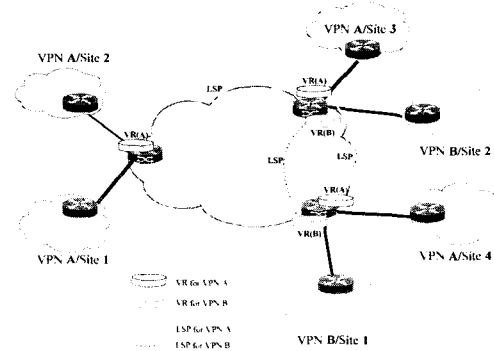
그림 3. VR을 이용한 네트워크 기반 MPLS VPN
