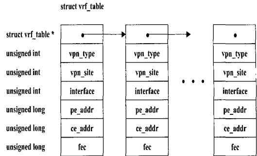
그림 6. /include/net/mpls.h 파일에 정의된 vrf_table 구조체
