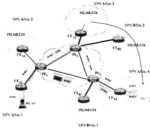
그림 1. MPLS VPN 구성 및 노드 이동 예
