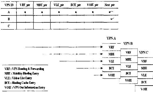
그림 5. VPN 인덱스 테이블
