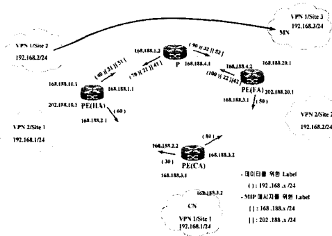
그림 8. 시험 환경 구성 및 레이블 분배 과정
