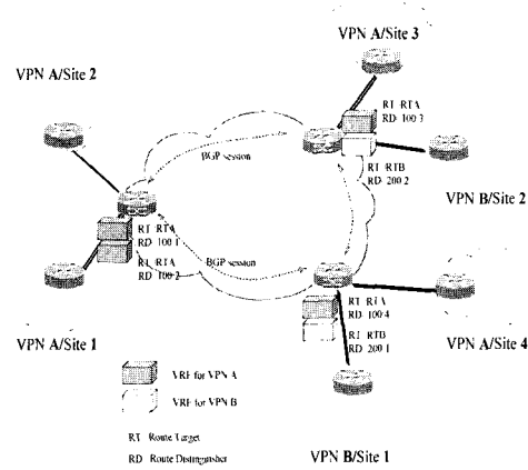
그림 2. BGP-E를 이용한 네트워크 기반 MPLS VPN
