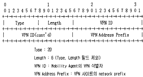
그림 4. ICMP Agent Advertisement 메시지 내의 VPN Information Extension
