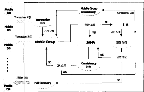
<그림 3> 시물레이션 프로세스
