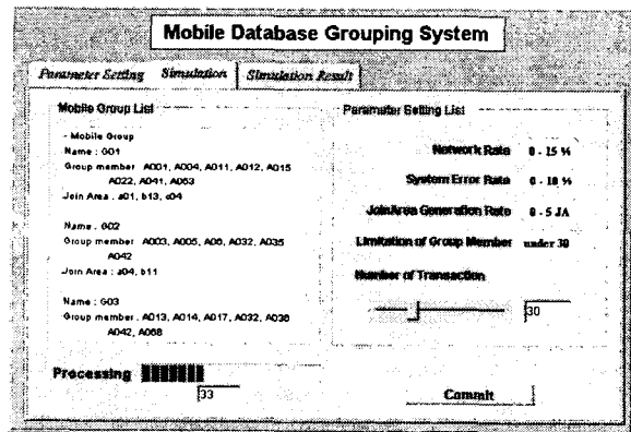
<그림 5> 시뮬레이션 인터페이스
