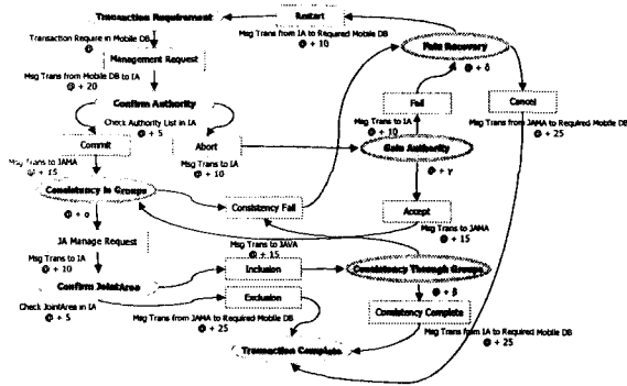
<그림 4> Hierarchical Extended Petri Net
