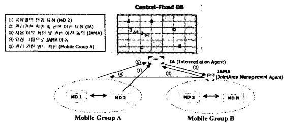
<그림 2> 공유영역 관리 메카니즘 개요도
