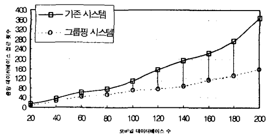
<그림 6> 기존 시스템과 그룹핑 시스템 시뮬레이션
