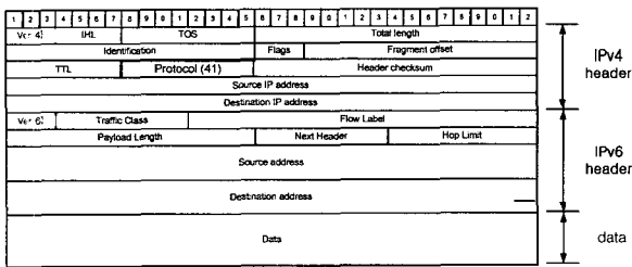
(그림 3) 터널링 패킷 IP 헤더
