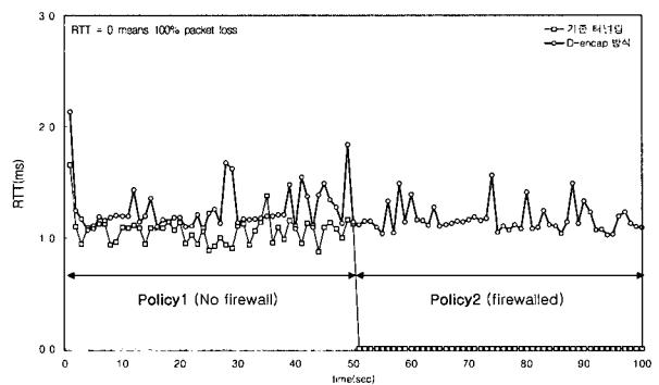
(그림 17) 기존 터널링과 D-encap 방식 비교
