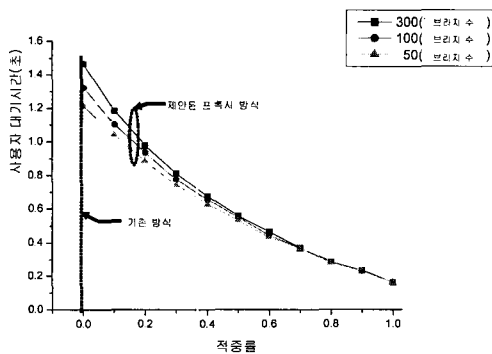
그림 12. 적중률에 따른 사용자 인증 대기시간
