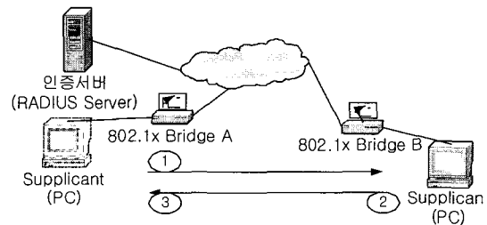
그림 8. 사용자 ID정보는 있으나 비밀번호가 일치 하지 않을 경우 발생 예
