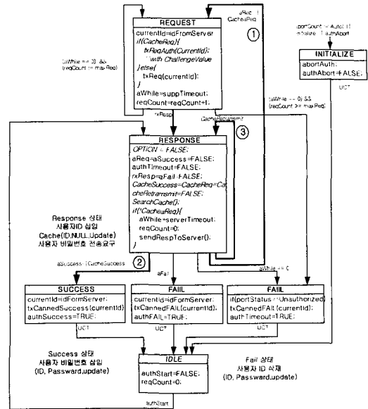
그림 3. 사용자 인증처리가 가능한 backend authentication의 상태도
