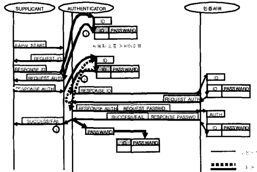
그림 9. 사용자 ID정보가 있으나 비밀번호가 일치 하지 않을 경우의 동작과정(제안방식)
