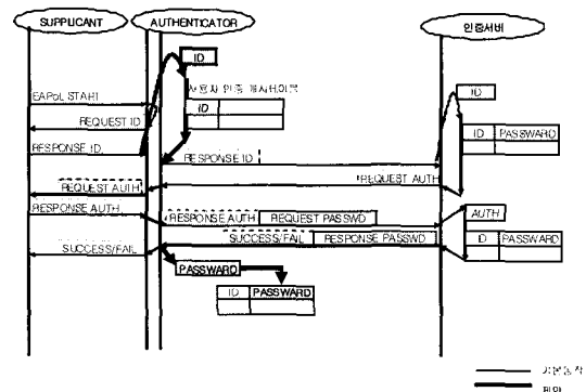
그림 6. 사용자 정보가 캐시테이블에 없는 경우의 동작과정(기존방식)
