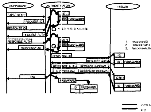
그림 7. 사용자 정보가 브리지 캐시테이블에 있는 경우의 동작과정(제안방식)
