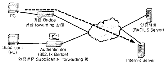
그림 1. 기존 LAN시스템과 IEEE802.1x 시스템의 구성비교
