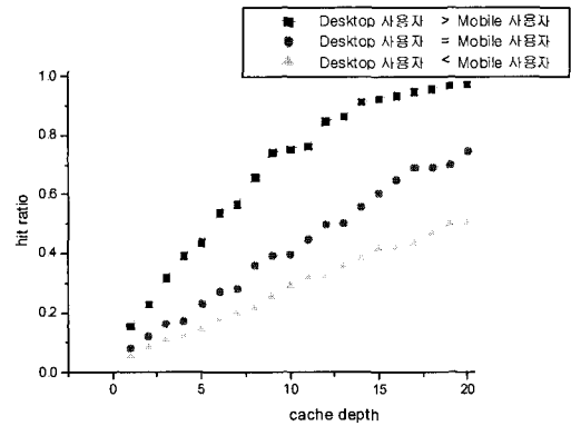
그림 10. 캐시테이블 크기에 따른 사용자의 적중률(사용자수 20)
