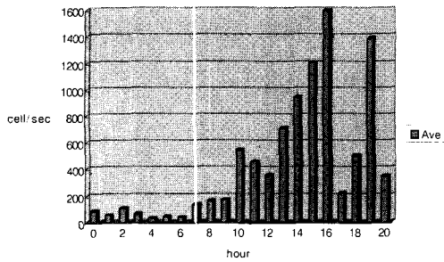
그림2. VPI=112, VCI=64회선의 측정 시간대별 트래픽 변화
