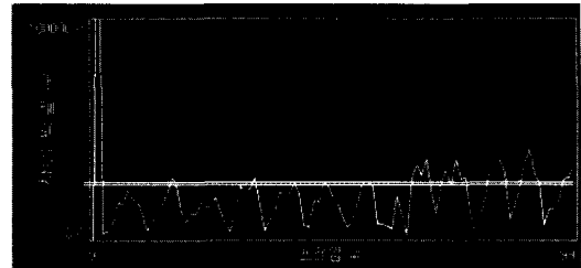
그림 4-2. 100 프레임에 대한 차이 픽셀 수와 프레임 수
