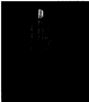
[차이 프레임]
