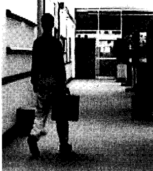
[분할될 프레임]
