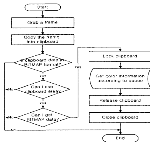
그림 7. 영상 획득의 흐름도 Fig. 7. The process for input image acquisition.
