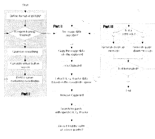
그림 2. 전체 시스템 흐름도 Fig. 1. System overview.
