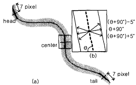
그림 2. 세션 영상을 이용한 선충의 두께 구하기 (a) 머리/꼬리와 중심의 두께 측정 부위, (b) 기울기
