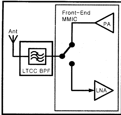
그림 1. WLAN RF 송수신기 Front End 모듈
