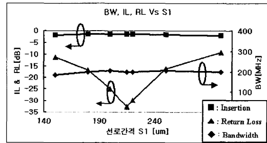
그림 7. 병렬결합 선로 간격 S1의 변화에 따른 여파기 특성
