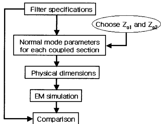
그림 2. 다층 병렬결합 구조의 LTCC 여파기 설계 절차
