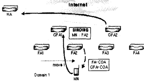
그림 1. MIPRR 기법에서의 영역내 이동 모델
