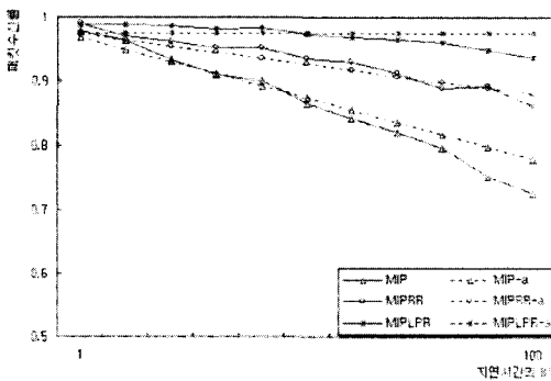
그림 15. 이동 노드와 HA의 거리에 따른 패킷 수신률
