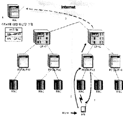
그림 5. MIPLPR 기법에서의 영역간 이동 모델
