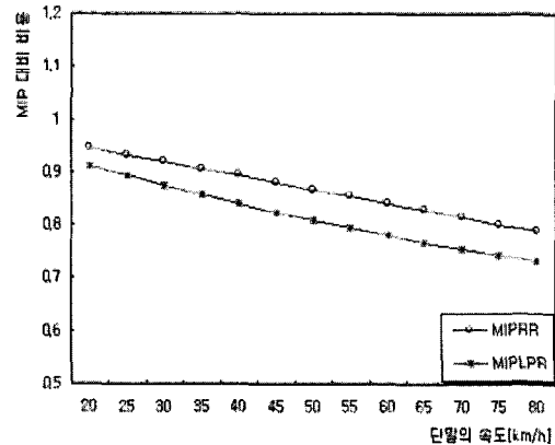
그림 7. 이동 노드의 속도에 따른 비용 비율
