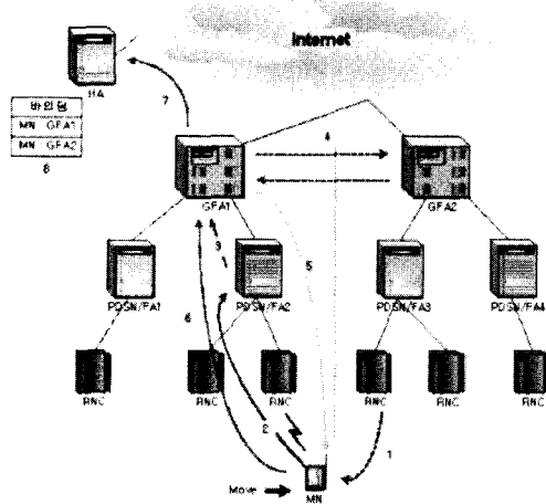
그림 4. MIPLPR 기법에서의 사전 등록 모델
