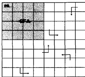
그림 11. 네트워크 환경
