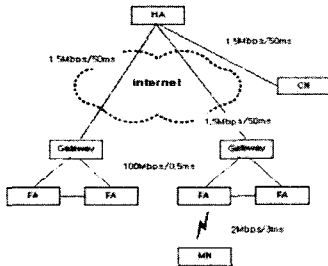
그림 10. 네트워크 모델
