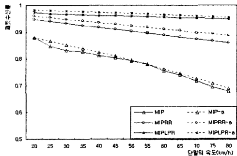
그림 13. 이동노드(차량)의 속도에 따른 패킷 수신률
