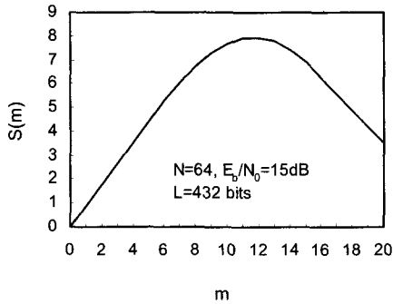
그림 1. 동시 전송 단말기 수별 성공 단말기 수
