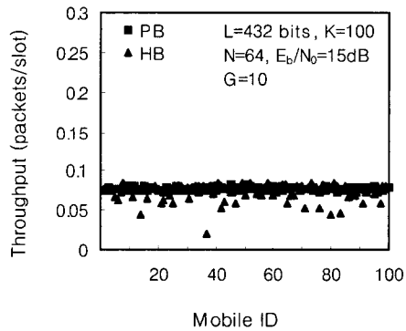
그림 10. 단말기별 처리율 ( G=10 )
