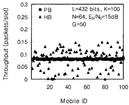
그림 11. 단말기별 처리율 ( G=50 )
