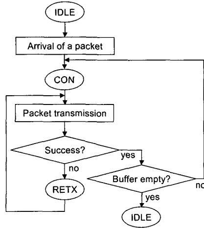
그림 2. 단말기의 동작 상태
