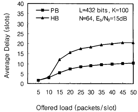
그림 9. 부하에 따른 평균 전송 지연 비교
