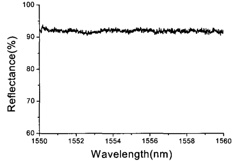
그림 4. 광섬유에 증착된 Cr/Au 박막의 반사 스펙트럼
