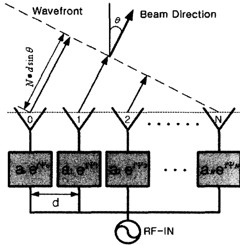
그림 1. TTD를 이용한 PAA 구조
