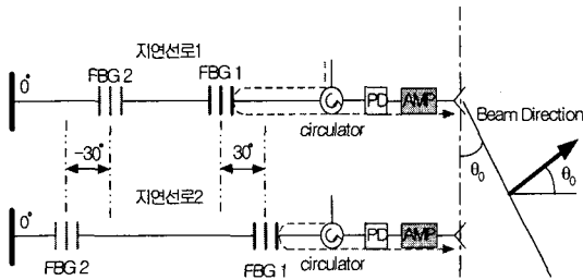
그림 3. 10 GHz 선형 PAA용 TTD
