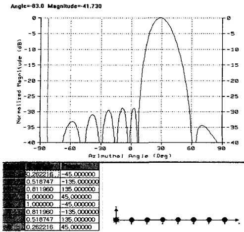
그림 9. 주사각이 30°인 경우 1-D 배열 계수의 시뮬레이션 결과
