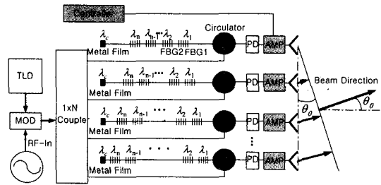
그림 2. 제안된 TTD의 구조
