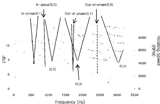
그림 3 회전속도변화에 따른 HDD 스핀들시스템의 고유진동 변화
