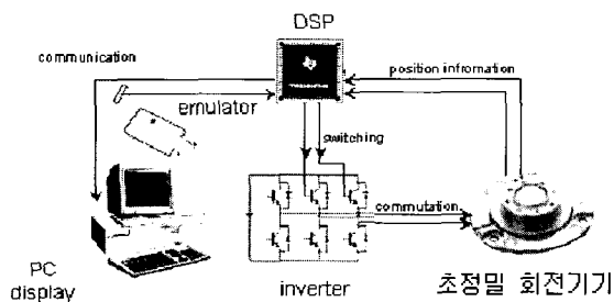
그림 5 초정밀 회전기기 구동 및 모니터링 시스템
