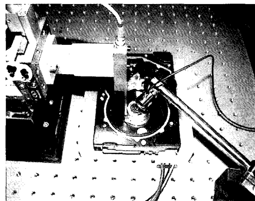
그림 4 초정밀 회전기기 진동 측정 시스템
