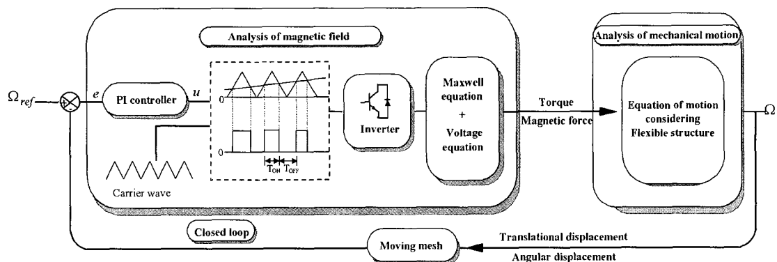
그림 6 초정밀회전기기 기전연성계 해석 흐름도
